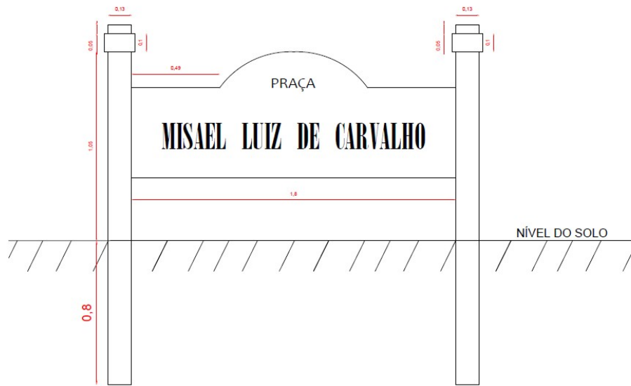
Figura 11 – PLACA DE MADEIRA MACIÇA
