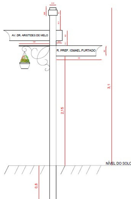
Figura 12 – POSTE DE IDENTIFICAÇÃO
