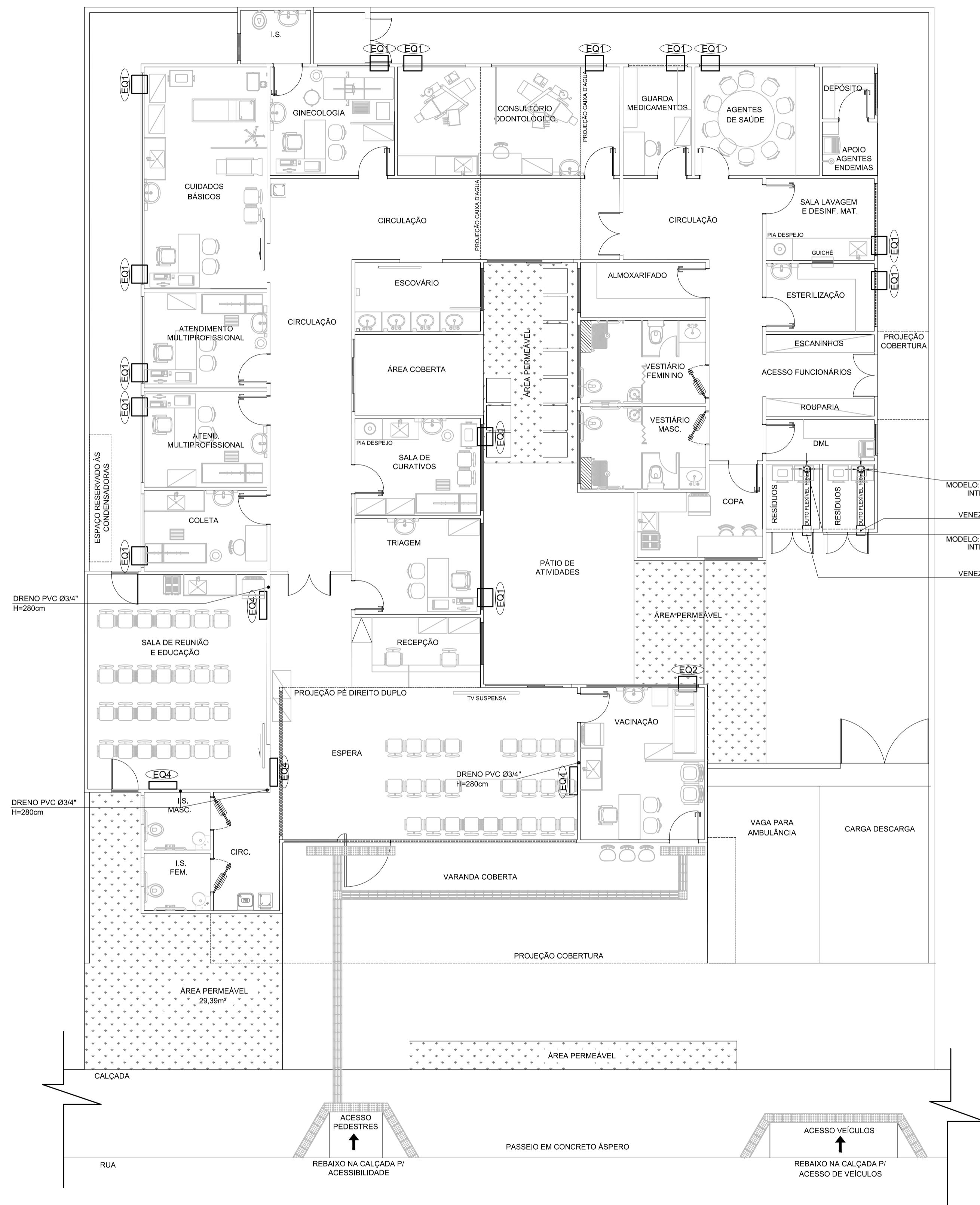
PLANTA DO TÉRREA ESCALA 1/75
